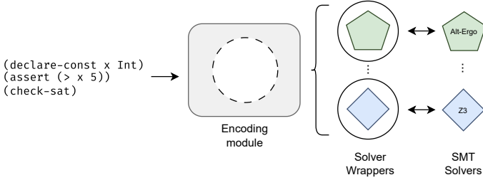
Fig. 3: The parametric Encoding module of SMT.ML.
